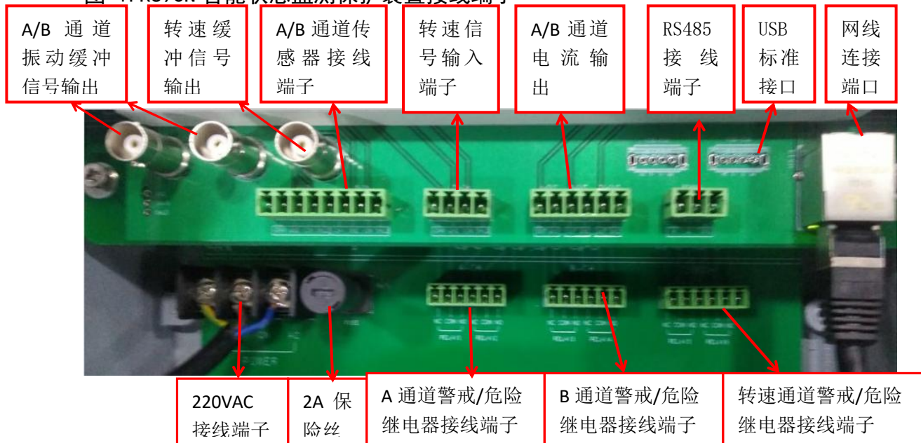
图 1. RS93N 智能状态监测保护装置接线端子
